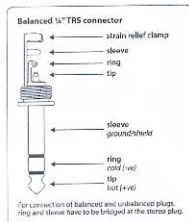
Fig. 3.3: Ficha jack estéreo de 6,3-mm
