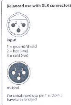
Fig. 3.1: Uniões XLR
