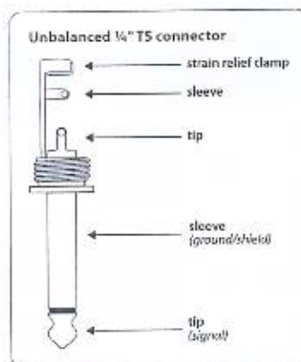
Fig. 3.2: Ficha jack mono de 6,3-mm
